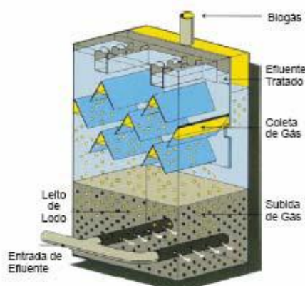
Figura 1: Esquema de um reator UASB.
