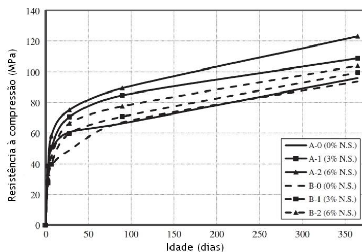
FIGURA 2: Evolução das resistências à compressão dos concretos.
