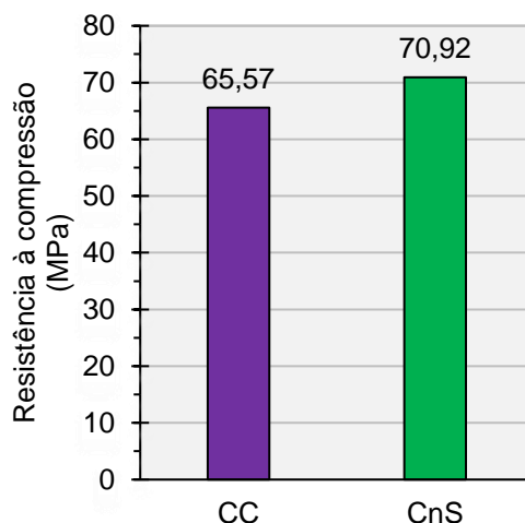
FIGURA 5: Resistência à compressão aos 28 dias.
