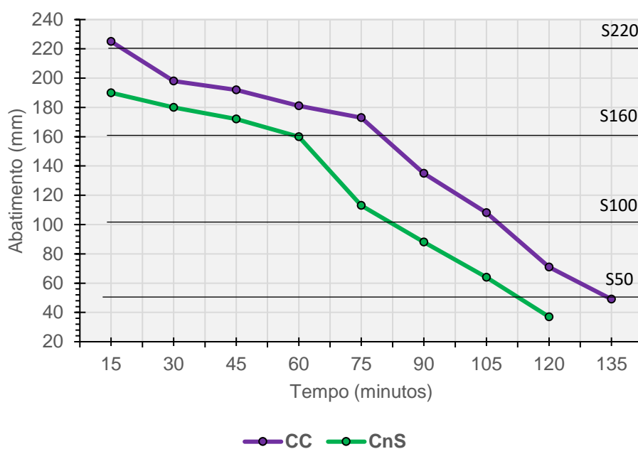
FIGURA 4: Evolução da consistência das misturas.
