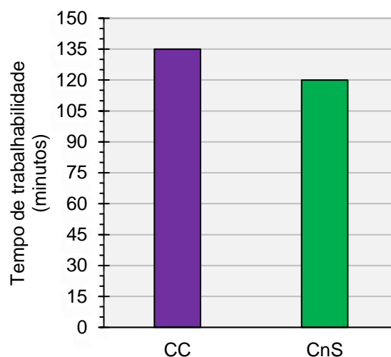
FIGURA 3: Tempo de trabalhabilidade das misturas. FONTE: Autoria própria.
