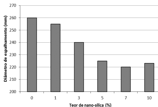
FIGURA 1: Fluidez de argamassas com diferentes teores de nS.
