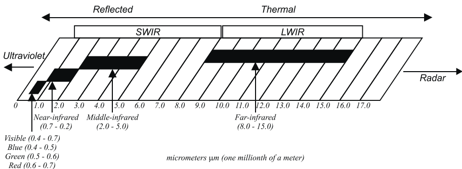
Figura 1: Espectro eletromagnético
