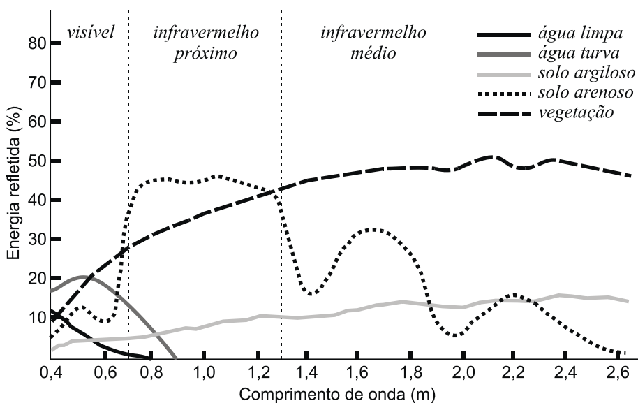
Figura 4: Curvas espectrais de diferentes alvos
