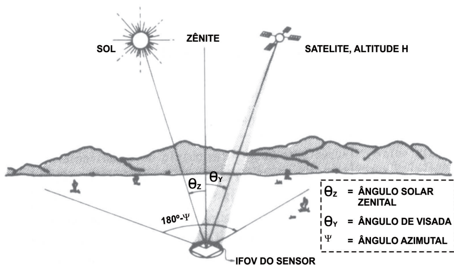
Figura 8: Variáveis da geometria de aquisição de dados que afetam as medidas de reflectância.
